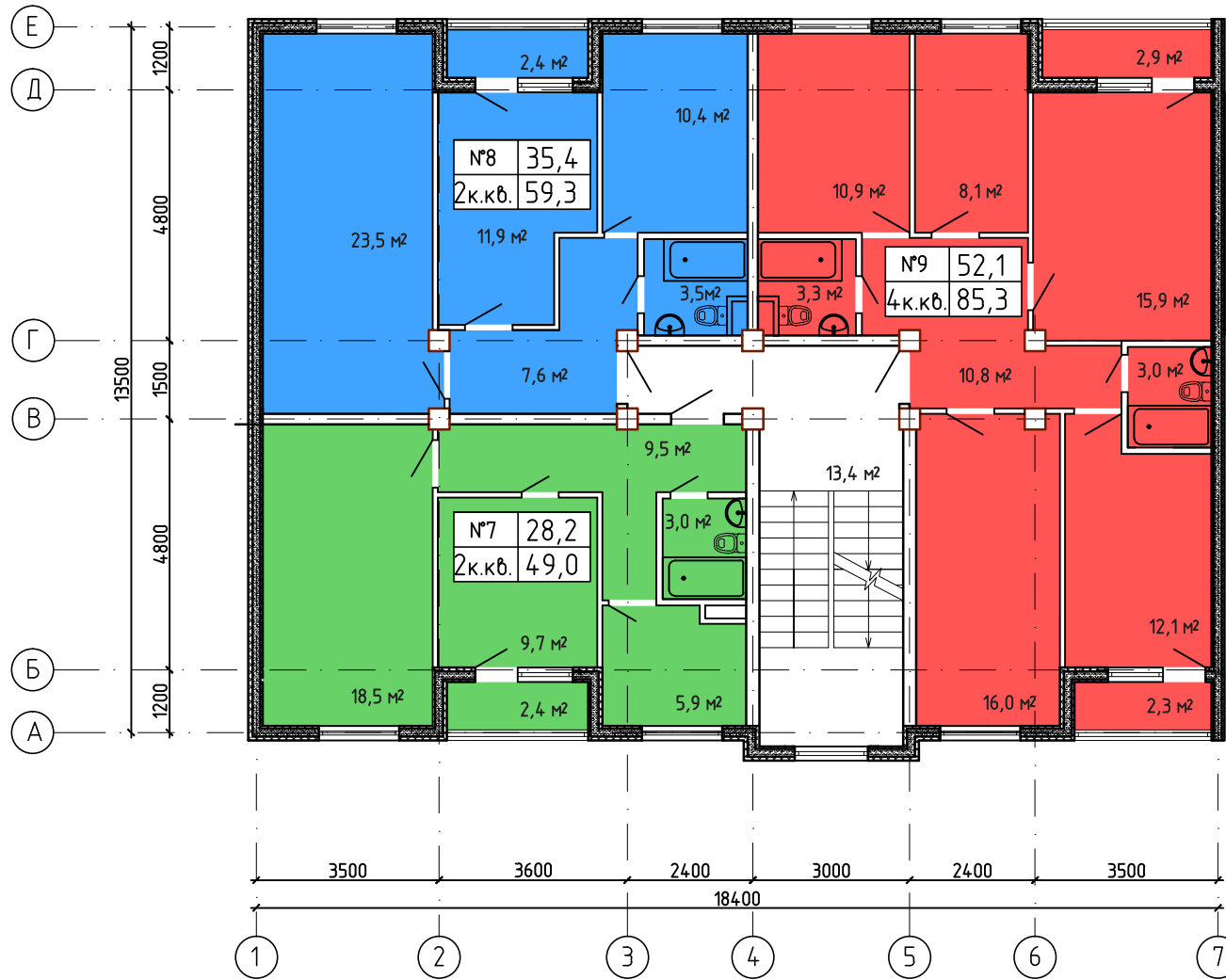
Компоновочная схема
