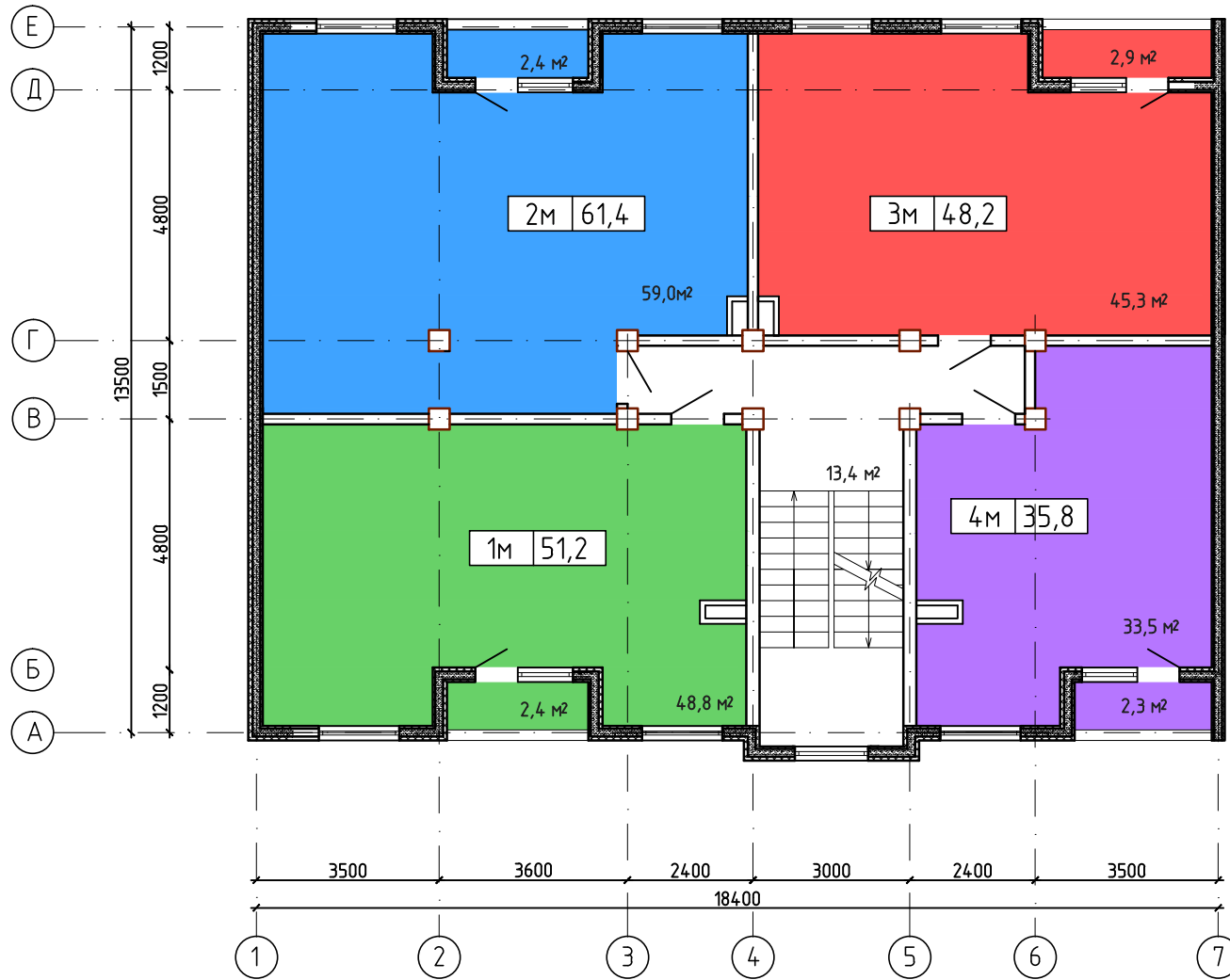
Компоновочная схема
