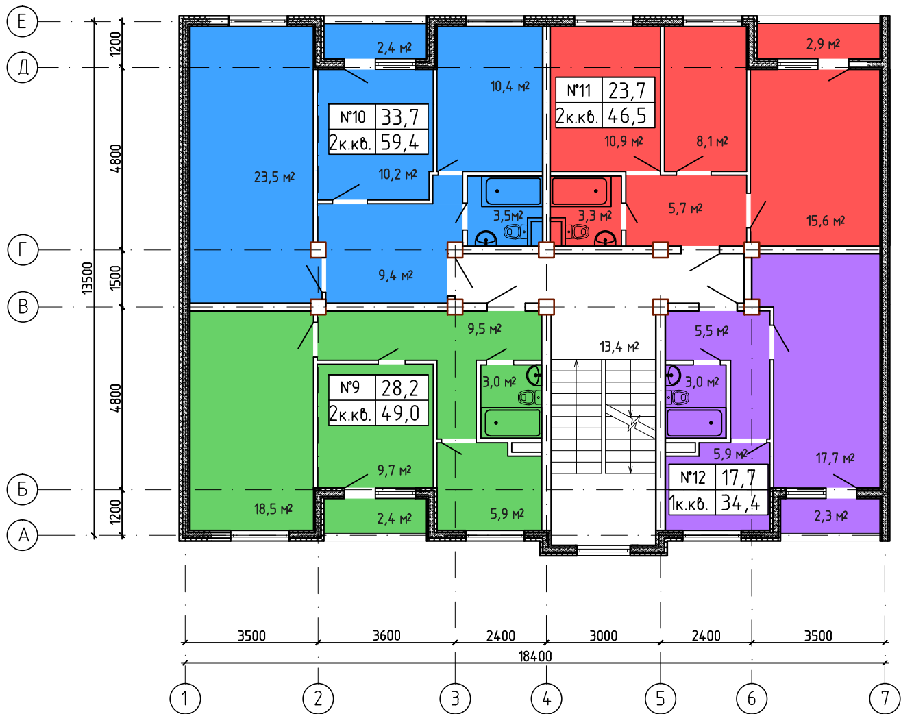
Компоновочная схема
