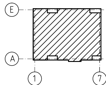
Компоновочная схема
